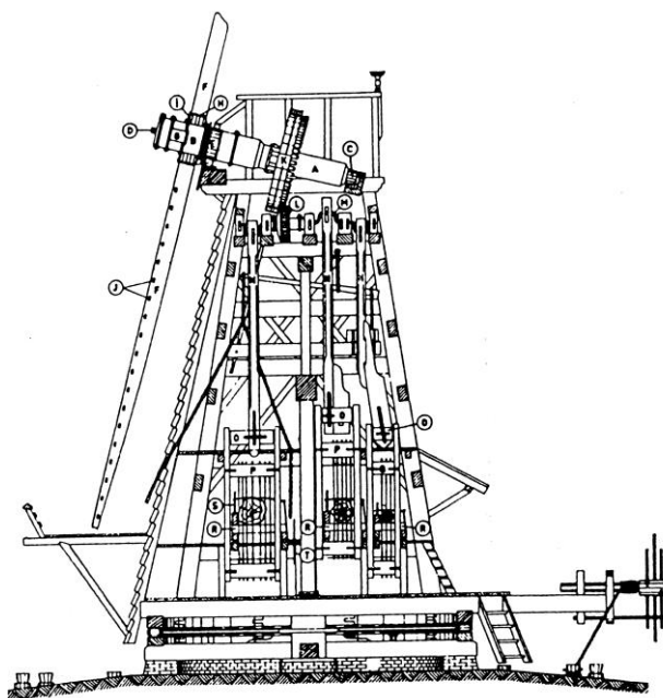
Doorsneden van de 'Zaanse' paltrok.
