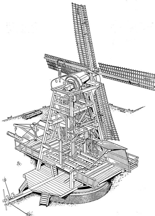
Perspectieftekening van de paltrok zaagmolen.
